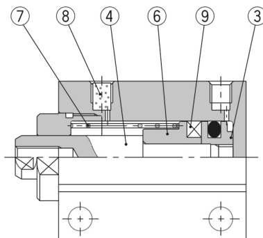
eingebauter Magnetring
