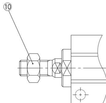
Kolbenstangen-Außengewinde
