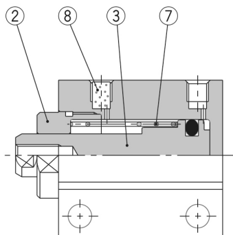
ohne Magnetring
