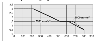
Vertikal/Spindelsteigung 10
